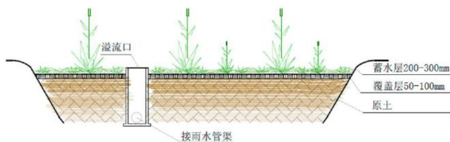
图 8.5.1（3）-1 简易型生物滞留设施典型构造示意图
