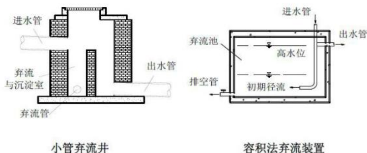
图 8.5.3 (2) 初期雨水弃流设施示意图
