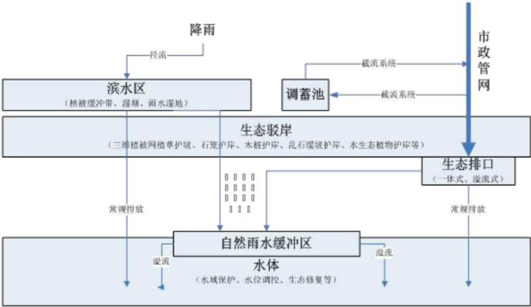
图 7.4.7 城市水系海绵措施衔接关系图
