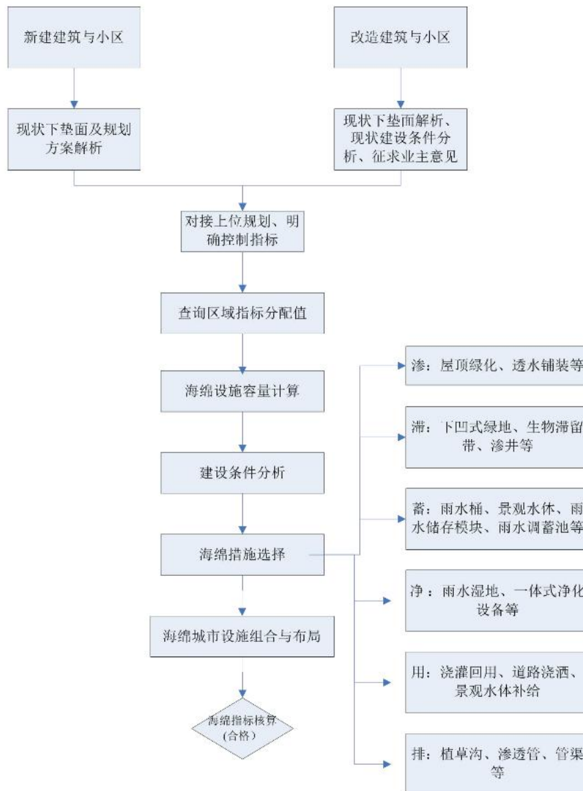
图 7.1.2 建筑与小区海绵性设计流程图
