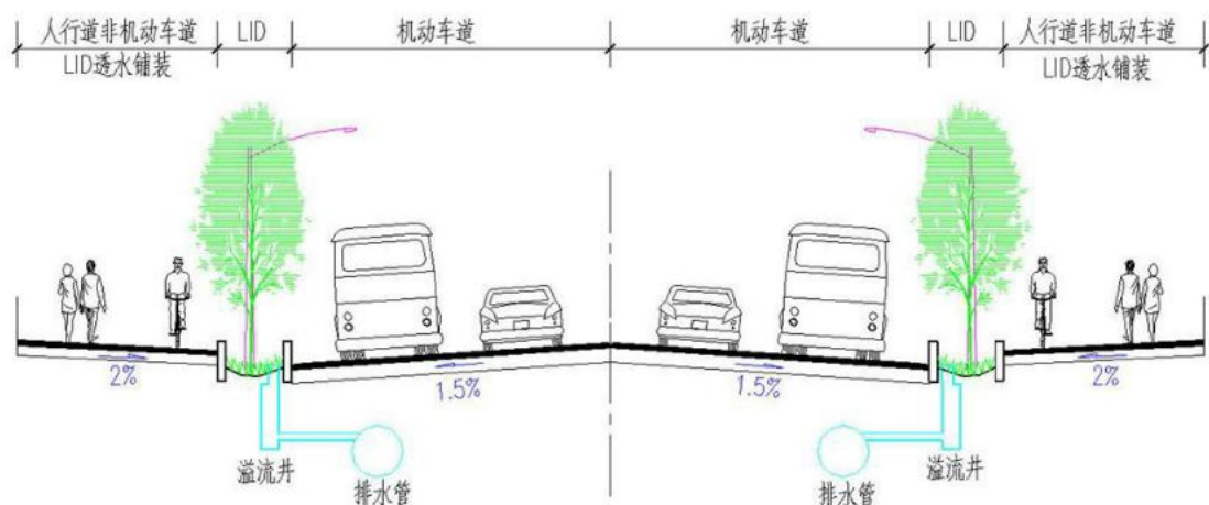
图 7.2.11 (1) 城市道路海绵性设计典型断面示意图
