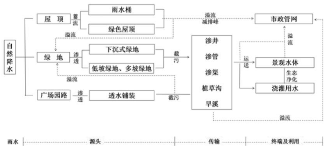
图 7.3.5 城市绿地与广场海绵措施衔接关系图
