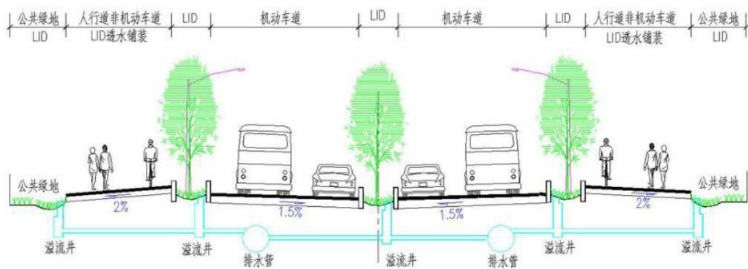
图 7.2.11 (4) 城市道路海绵性设计典型断面示意图
