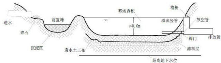
图 8.5.1 (4) -1 渗透塘典型构造示意图
