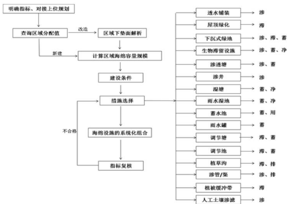
图 7.3.3 城市绿地与广场海绵性设计流程图
