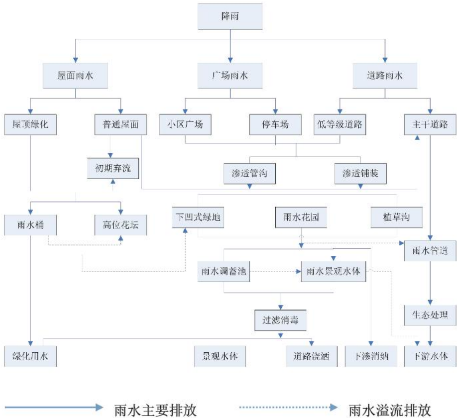
图 7.1.5 建筑与小区海绵措施衔接关系图
