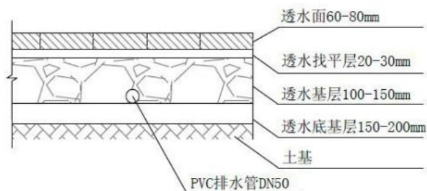
图 8.5.1（1）-1 透水砖铺装典型结构示意图
