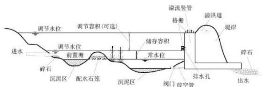
图 8.5.2(1) 湿塘典型构造示意图
