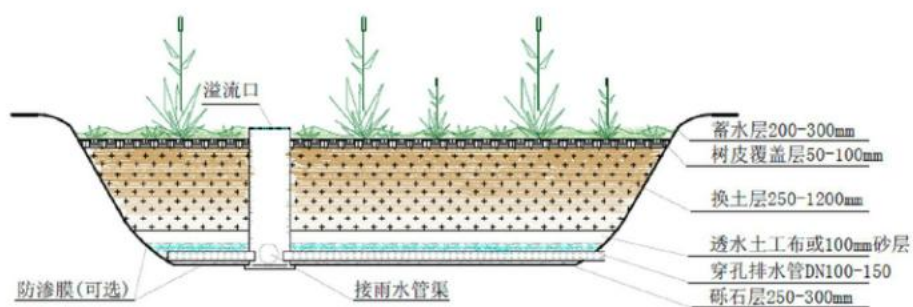
图 8.5.1 (3) -2 复杂型生物滞留设施典型构造示意图
