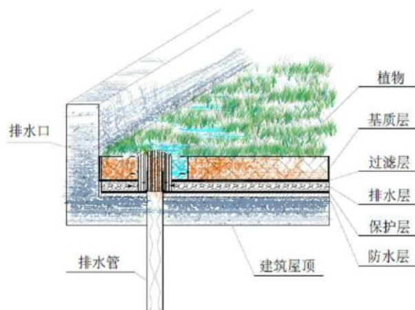
图 8.5.1 (2) -1 绿色屋顶典型构造示意图
