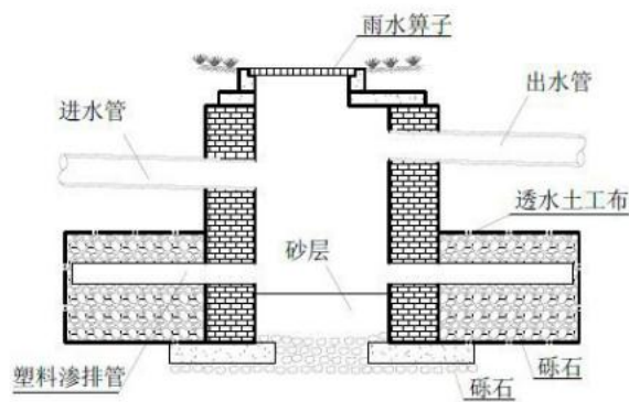
图 8.5.1(5) 辐射渗井的典型构造示意图
