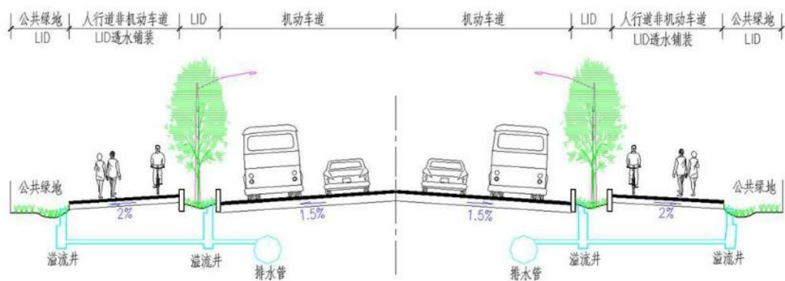
图 7.2.11 (2) 城市道路海绵性设计典型断面示意图
