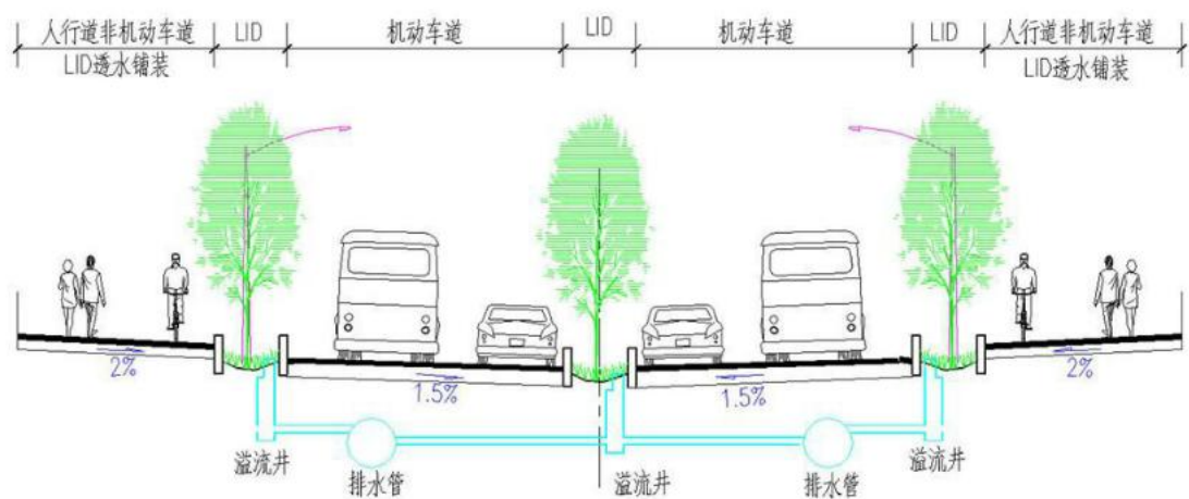
图 7.2.11 (3) 城市道路海绵性设计典型断面示意图
