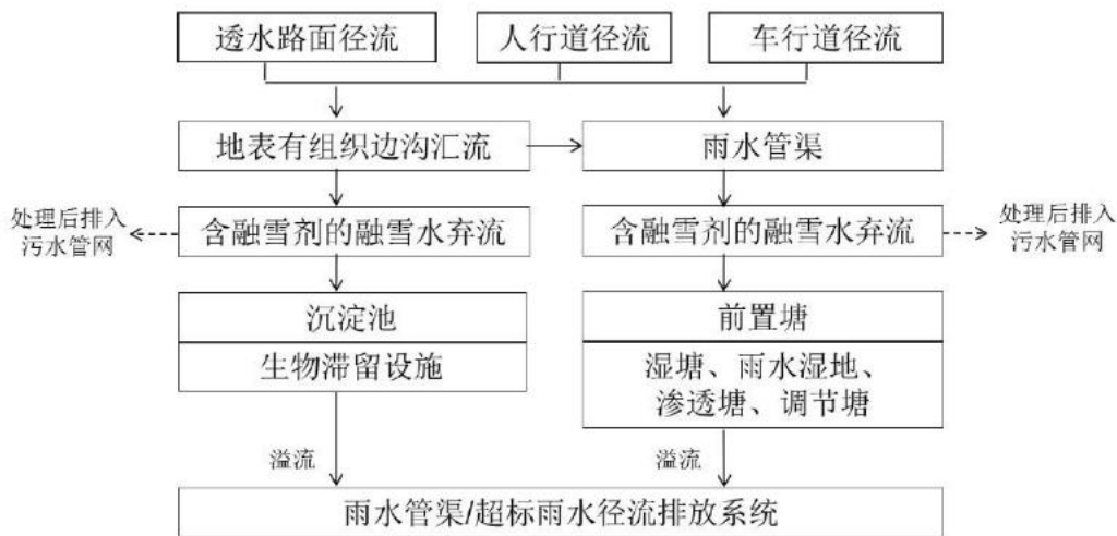
图 7.2.24 城市道路海绵措施衔接关系图
